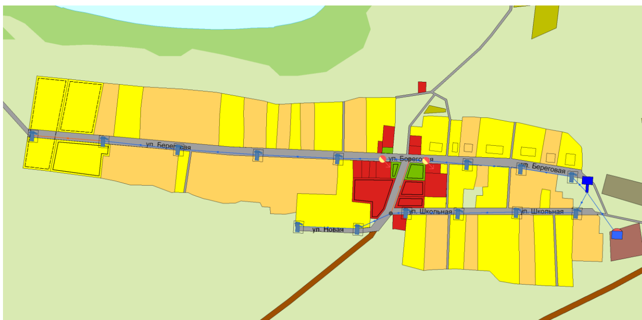
Рисунок 8 - Существующая схема водопроводной сети с. Кушаги
