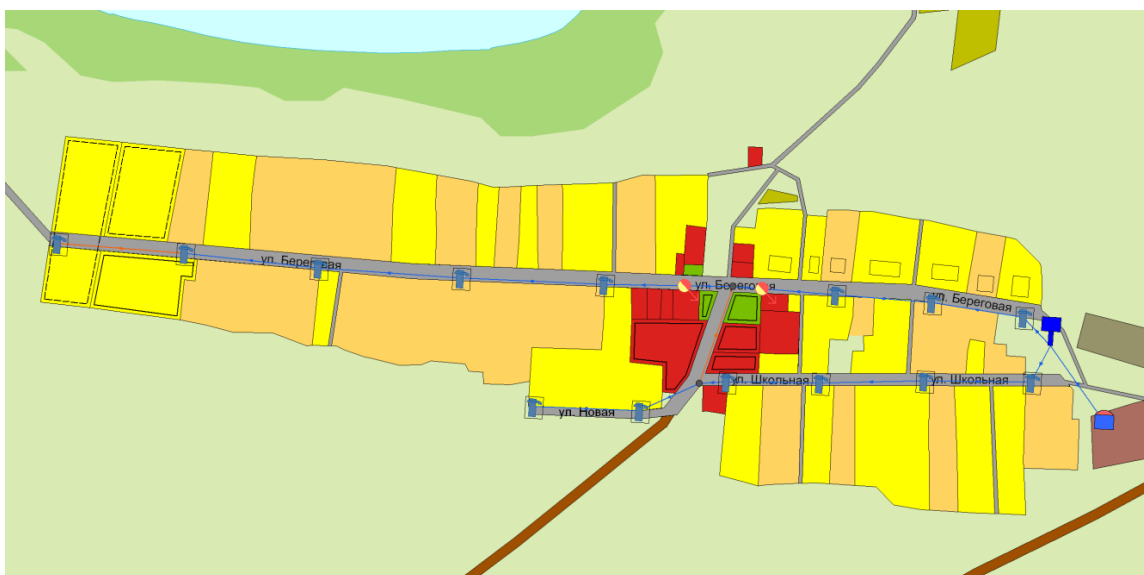
Рисунок 1 - Зона действия централизованного водоснабжения с. Кушаги
